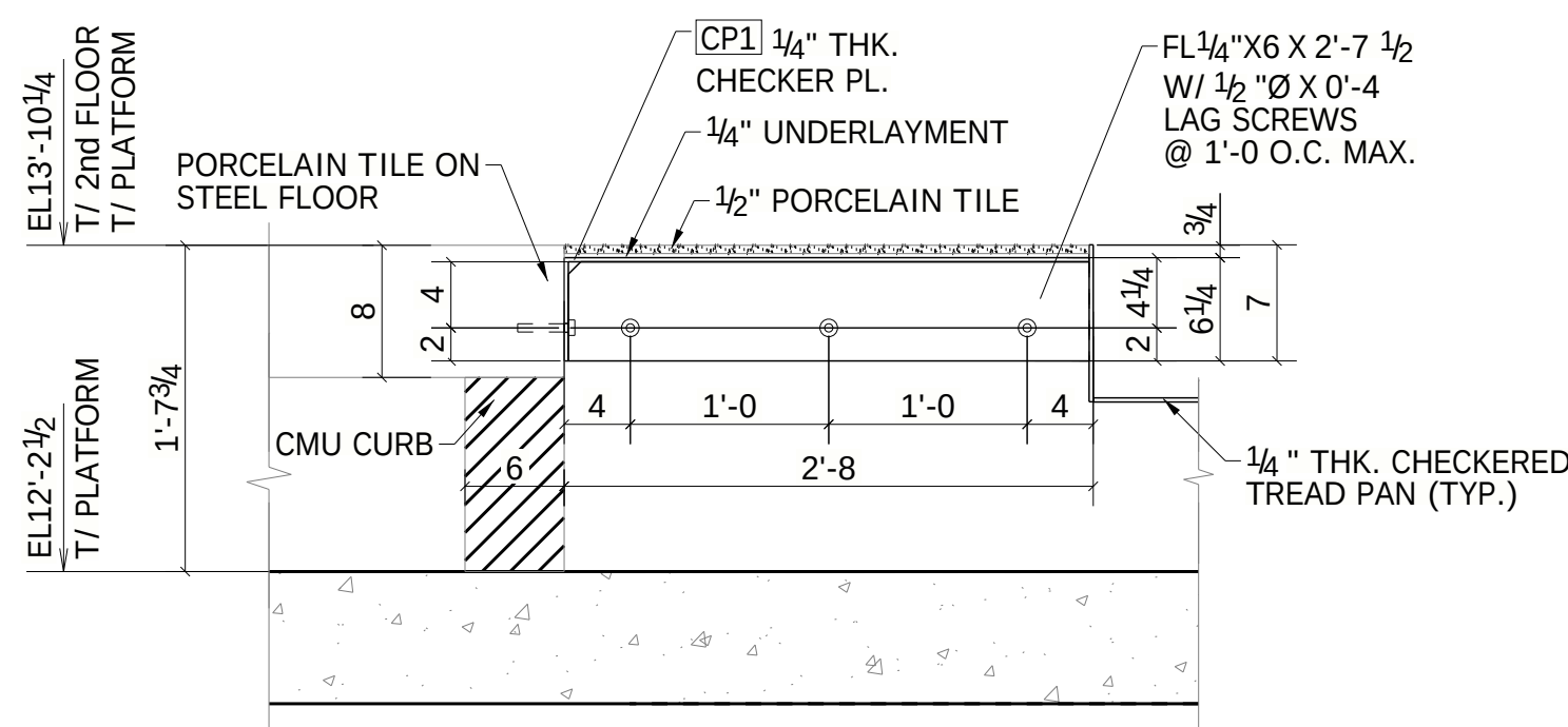
SECTION E - E ME1
