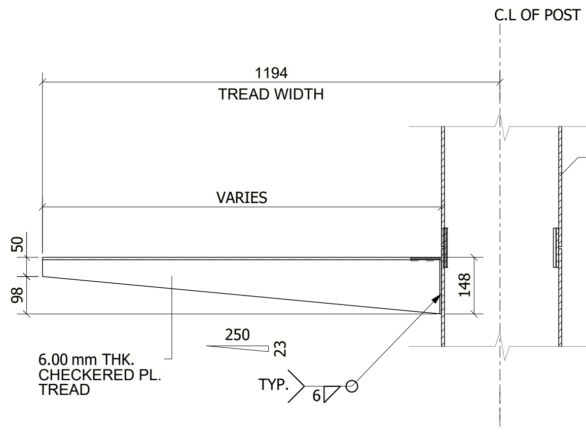
SECTION BB - BB
