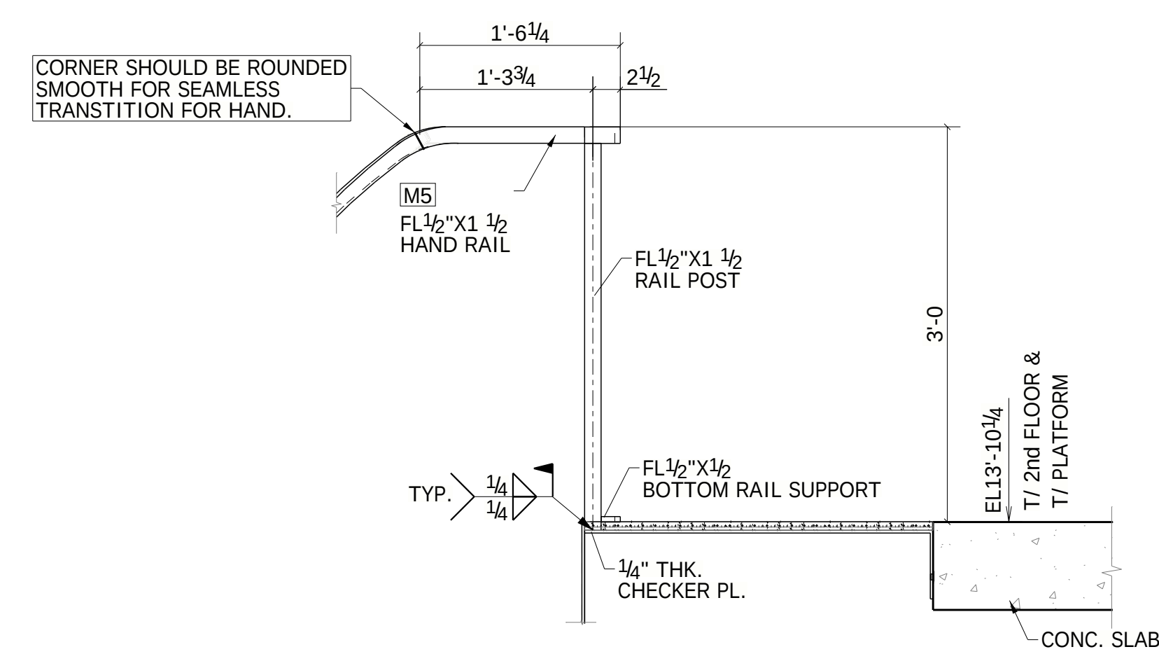
SECTION F - F ME1
