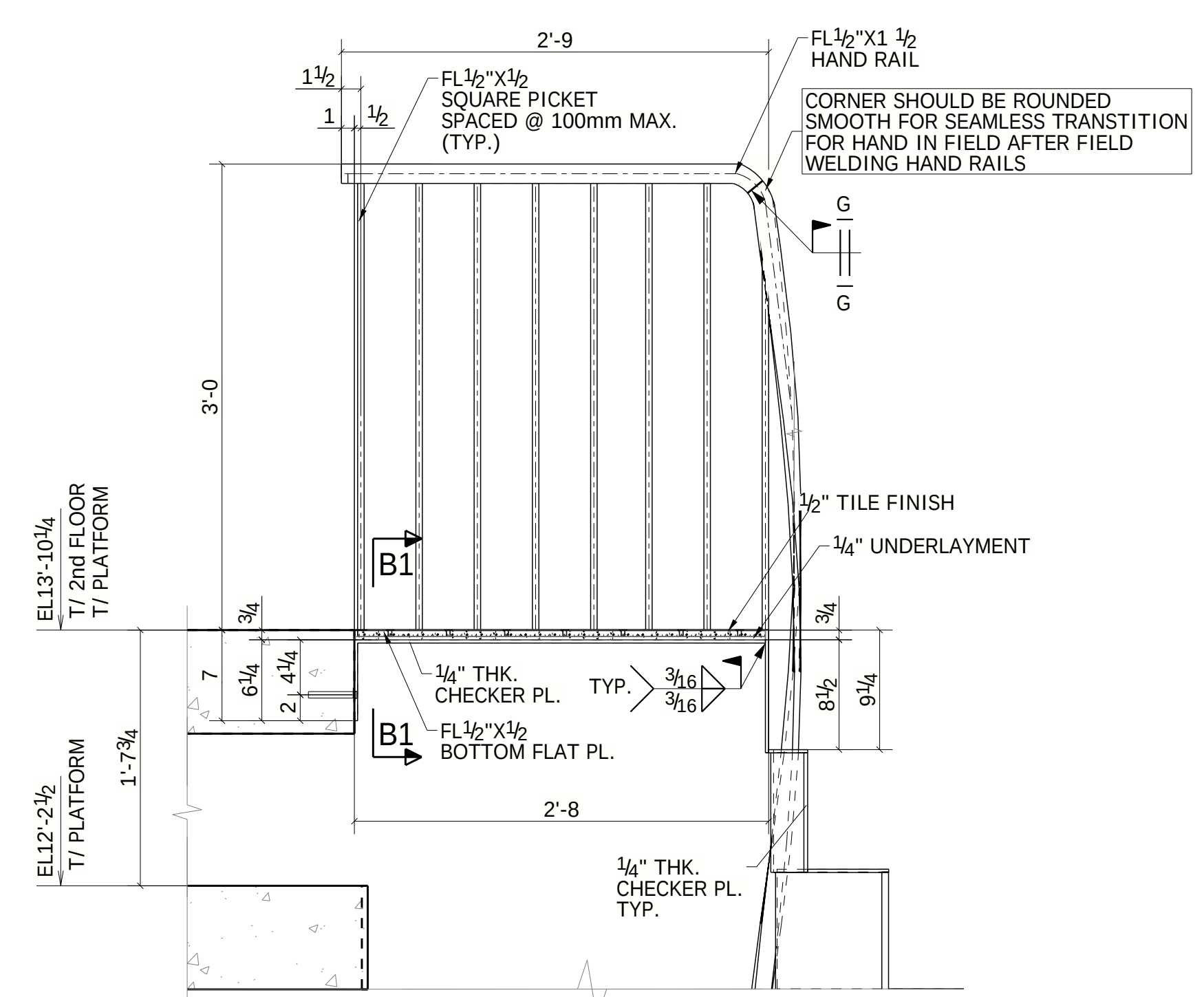
SECTION B - B ME1
