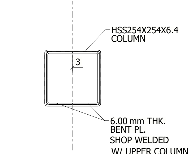
SECTION 3A - 3A
