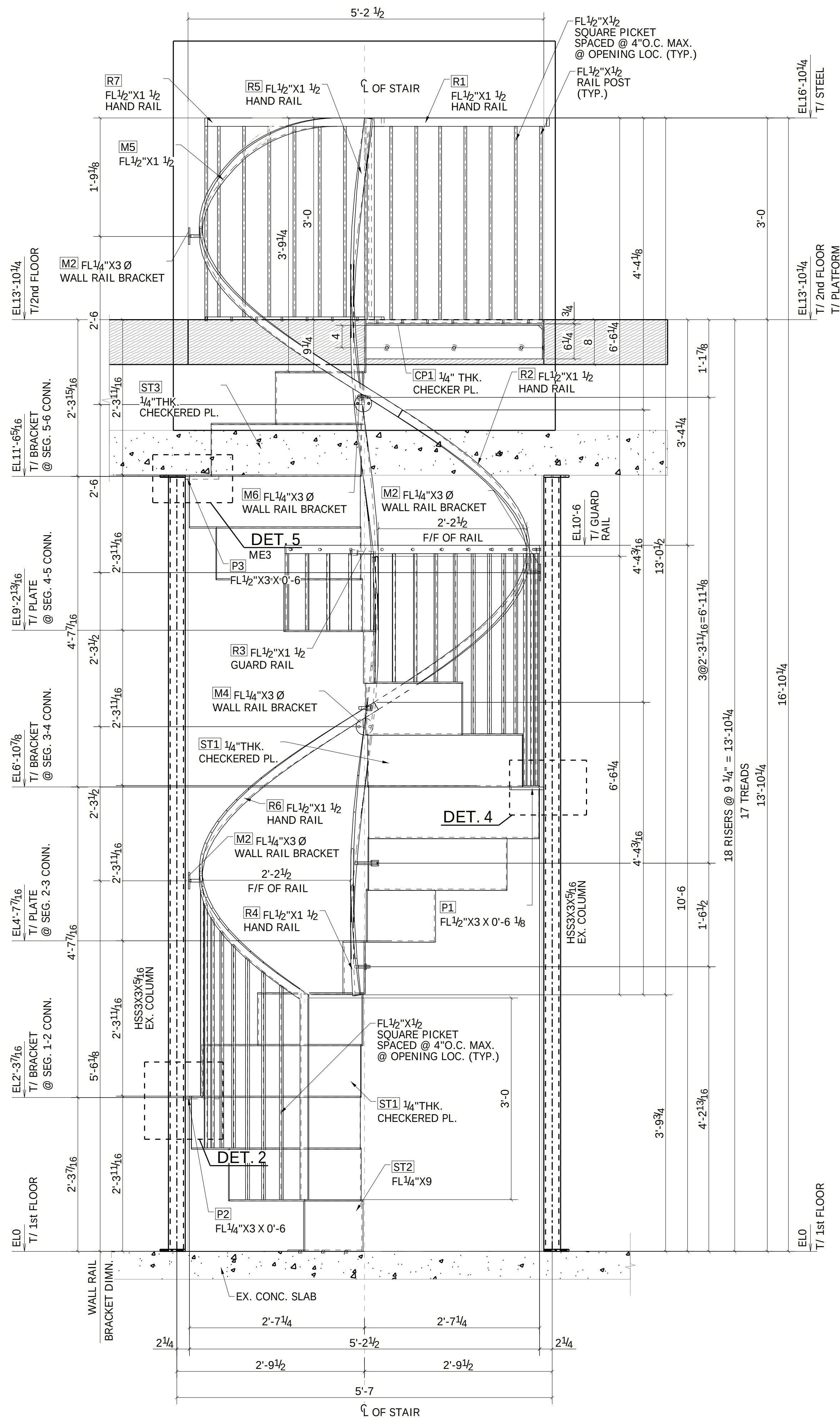
SECTION A - A ME1
