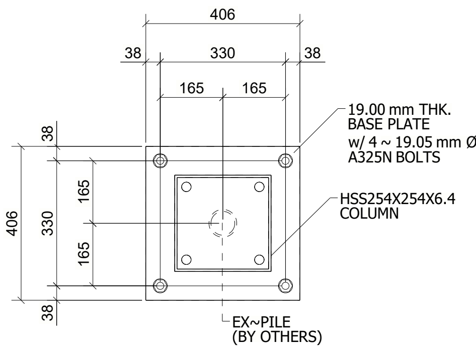
SECTION 1A - 1A
