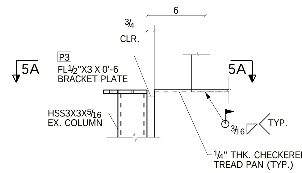
DETAIL 5 ME2
