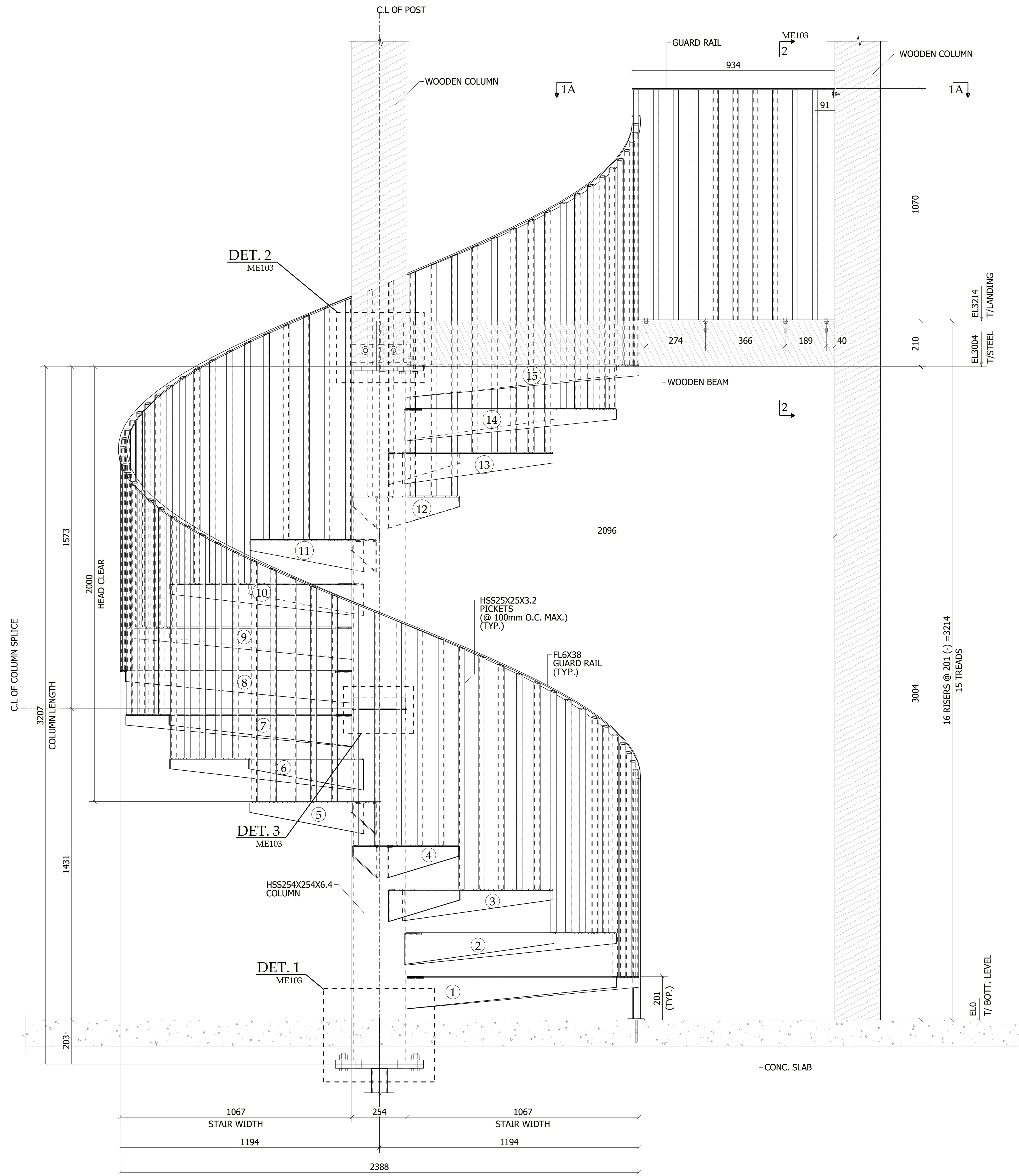
SECTION A - A ME101 (REFER : COUPE GENERALE C-C/ 351 )
