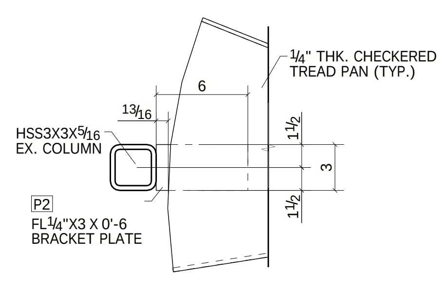
SECTION 2A - 2A
