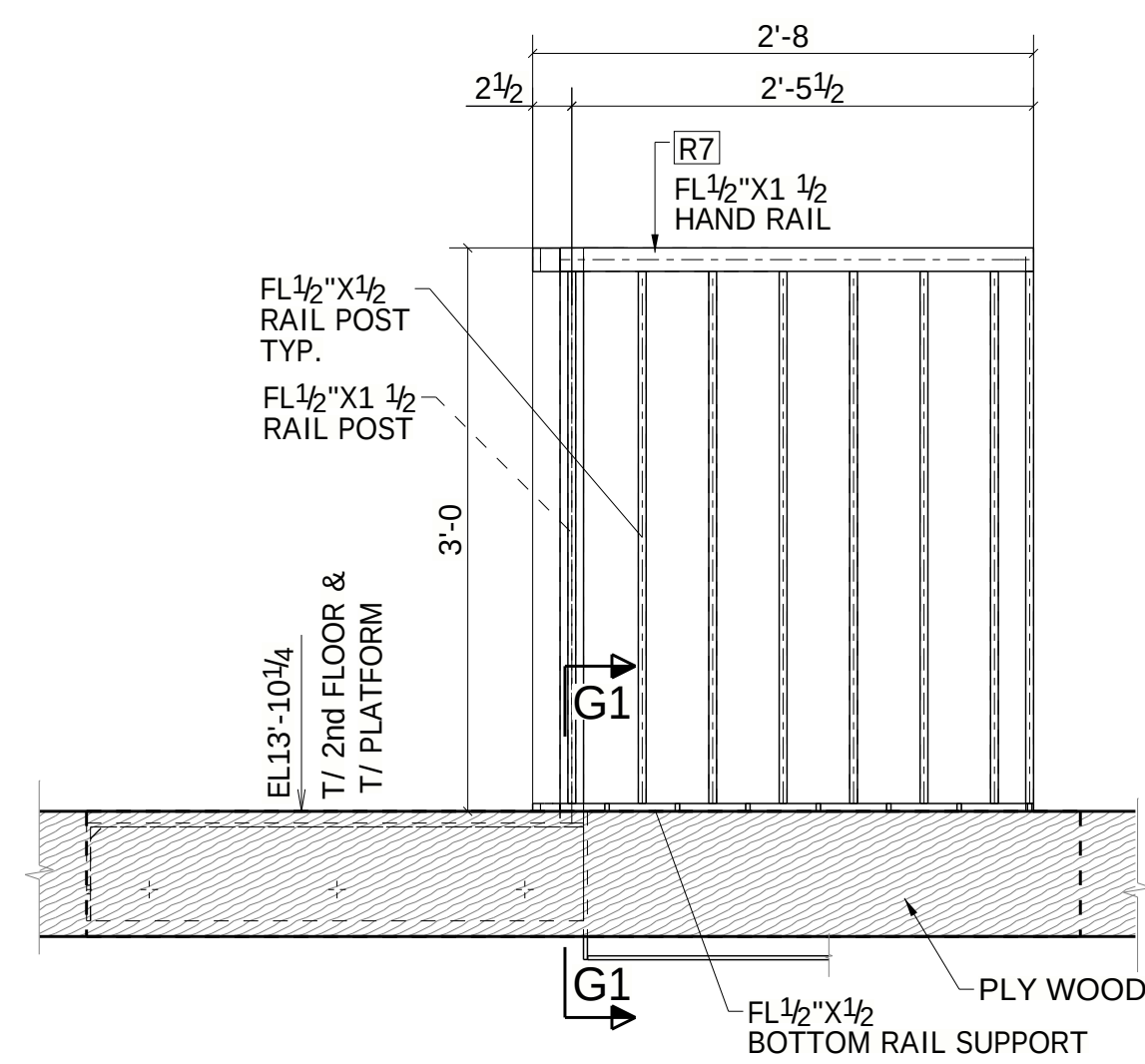
SECTION G - G ME1
