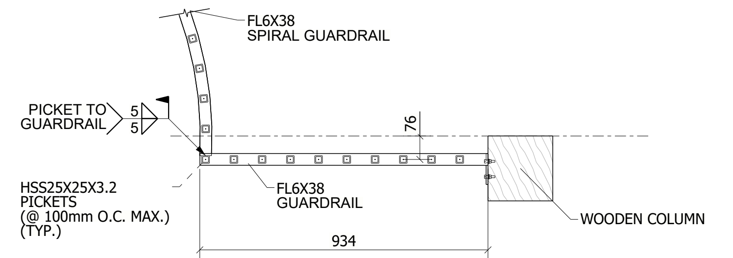
SECTION 1A - 1A
