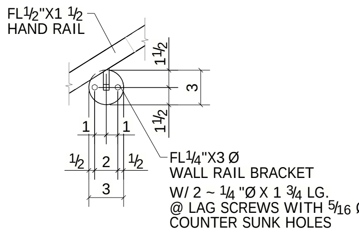
SECTION C1 - C1
