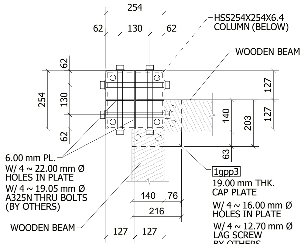
SECTION 2A - 2A
